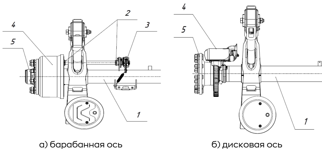
Рис. 2.5 - Оси
