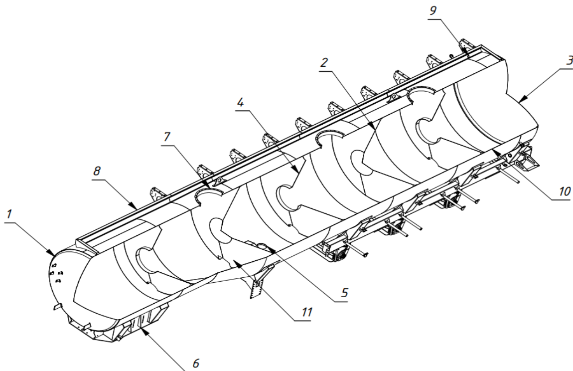
Рис. 2.3 – Цистерна полуприцепа
