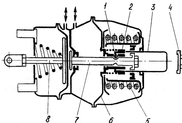
Рис. 2.16 – Тормозная камера с энергоаккумулятором
