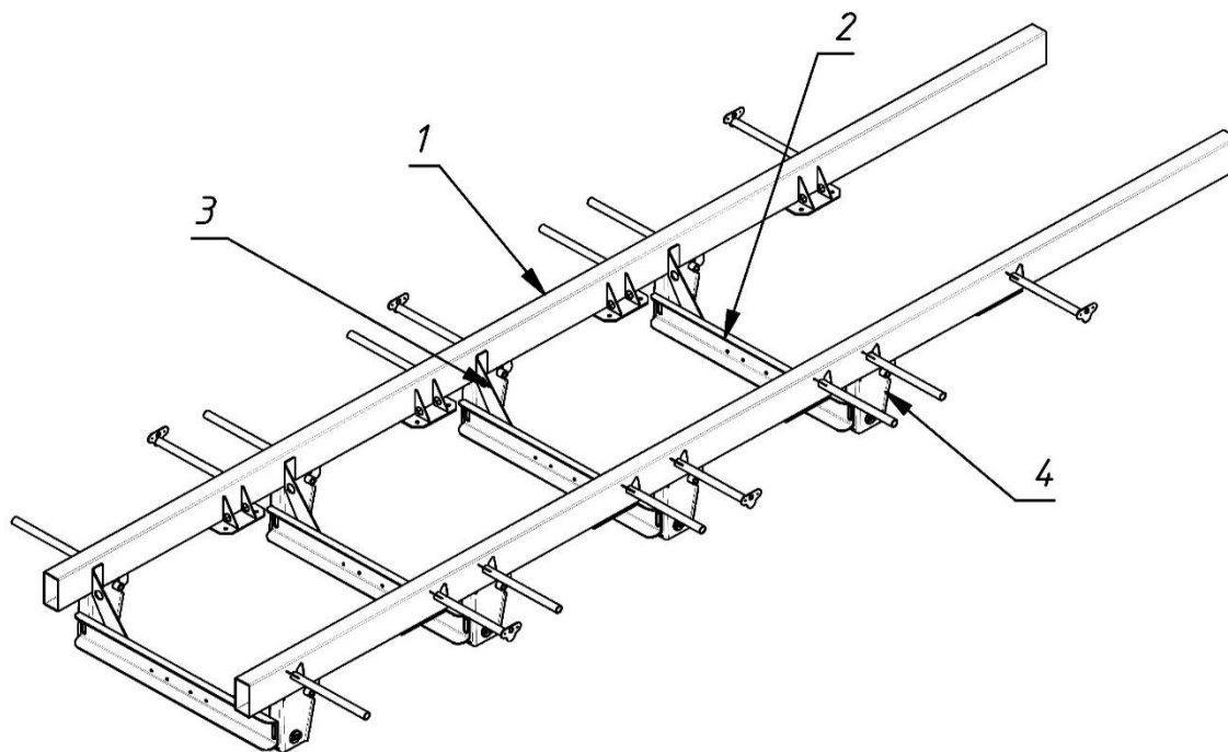
Рис. 2.4 - Рама полуприцепа
