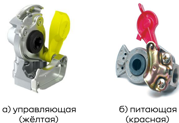
Рис. 2.13 – Соединительные головки
