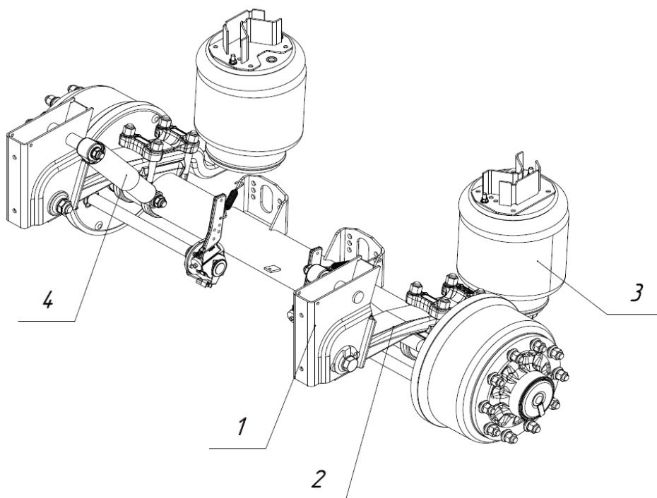
Рис. 2.6 - Осовой агрегат на пневмоподвеске
