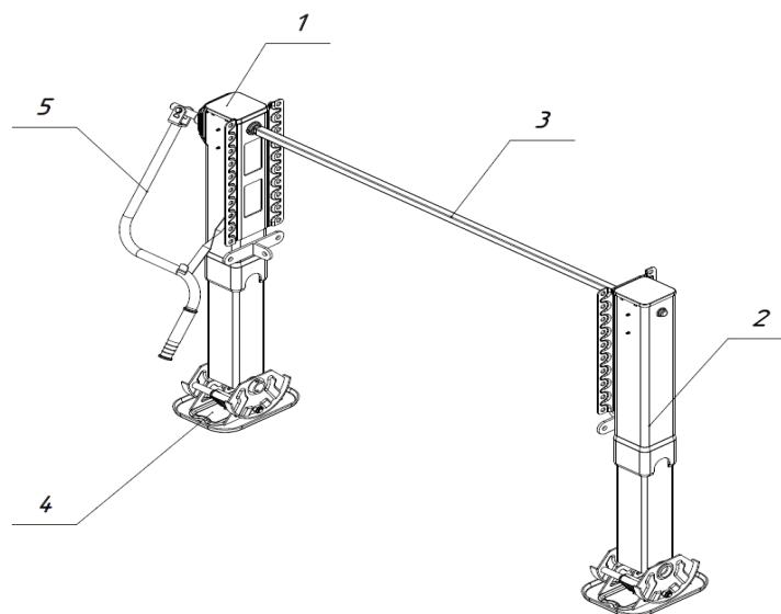
Рис. 2.12 – Опорное устройство
