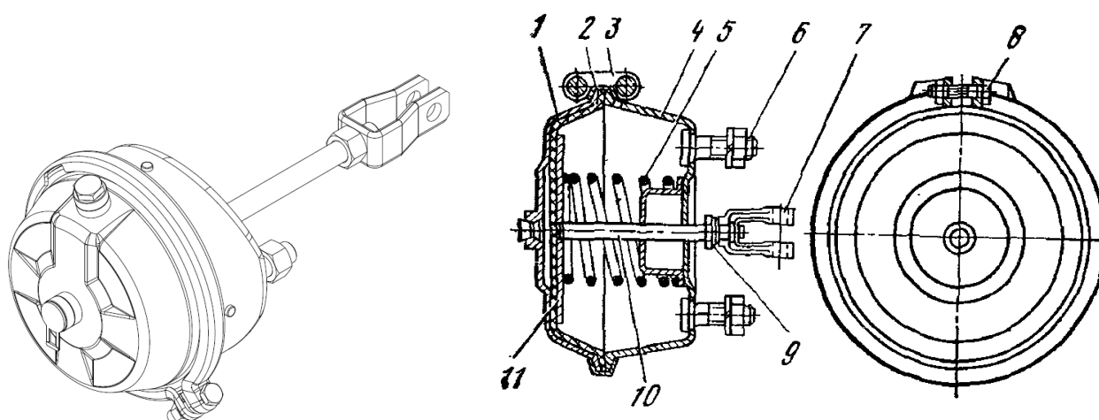
Рис. 2.21 – Тормозная камера
